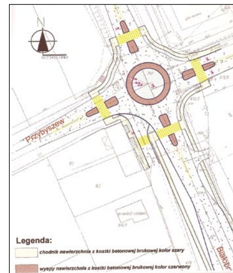
Projekt ronda w Fałęcicach zrealizowany został z inicjatywy Starostwa Powiatowego.
